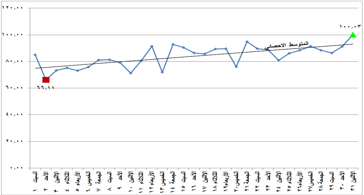
شكل (٢١) الطاقة الكهربائية المنتجة من المصادر غير الحرارية خلال شهر اغسطس ٢٠٢٠
