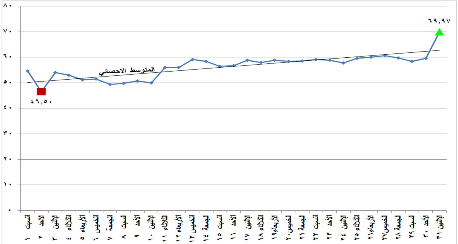
شكل (٢٣) الطاقة الكهربائية المنتجة من المصادر المائية خلال شهر أغسطس ٢٠٢٠
