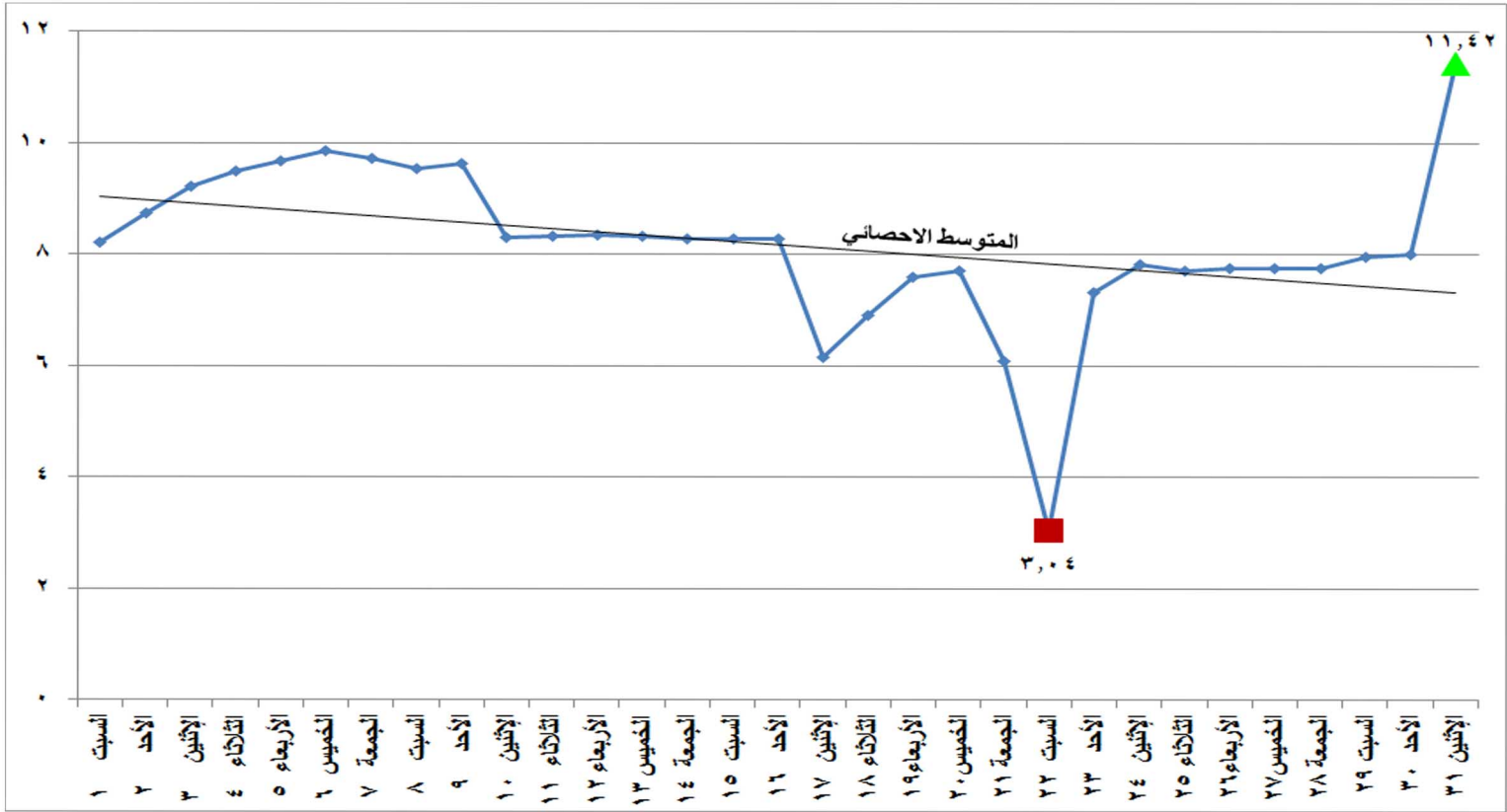
شكل (١٩) الطاقة الكهربائية المنتجة من المازوت خلال شهر أغسطس ٢٠٢٠
