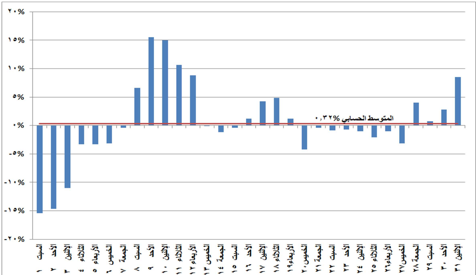
شكل (١٦) نسب التغير في الطاقة الكهربائية المنتجة خلال شهر أغسطس ٢٠٢٠ مقارنة بالشهر المماثل من العام السابق
