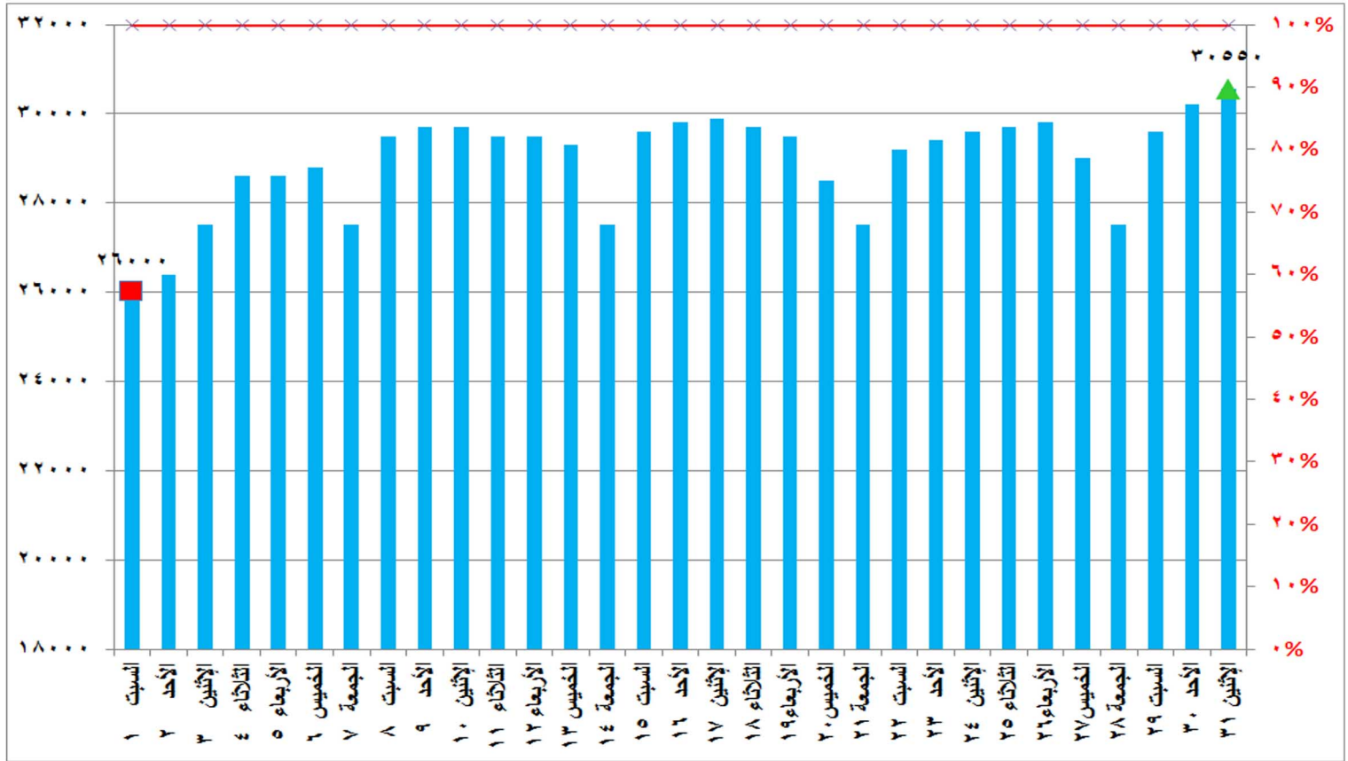
شكل (٥) قدرات الانتاج المتاحة ونسبتها للحمل الأقصى خلال شهر أغسطس ٢٠٢٠
