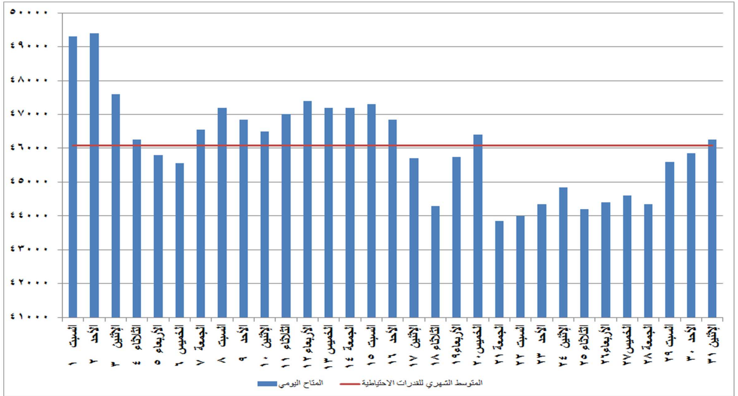
شكل (٢٧) القدرات المتاحة يوميا والمتوسط الشهري للقدرة الاحتياطية خلال شهر أغسطس ٢٠٢٠
