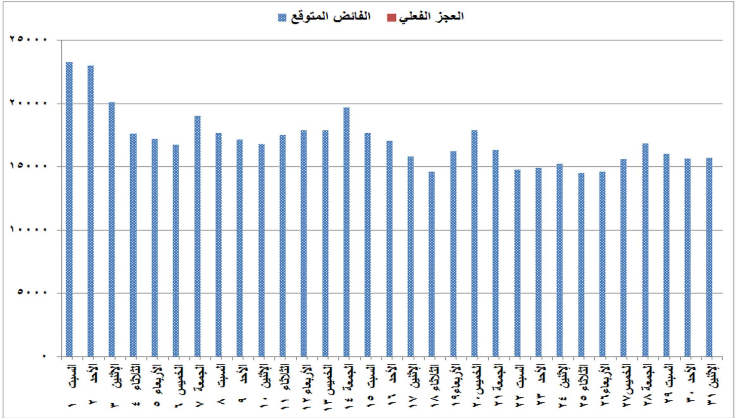
شكل (٧) الفائض والعجز المتوقع للقدرات خلال شهر أغسطس ٢٠٢٠
