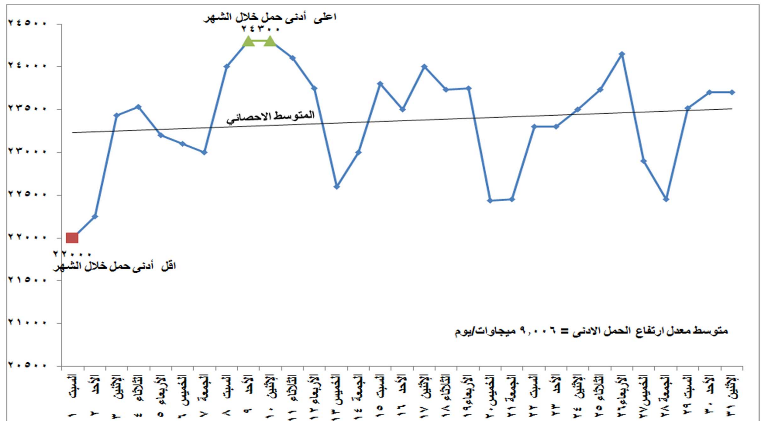
شكل (٢) تطور الحمل الادنى اليومي خلال شهر اغسطس ٢٠٢٠
