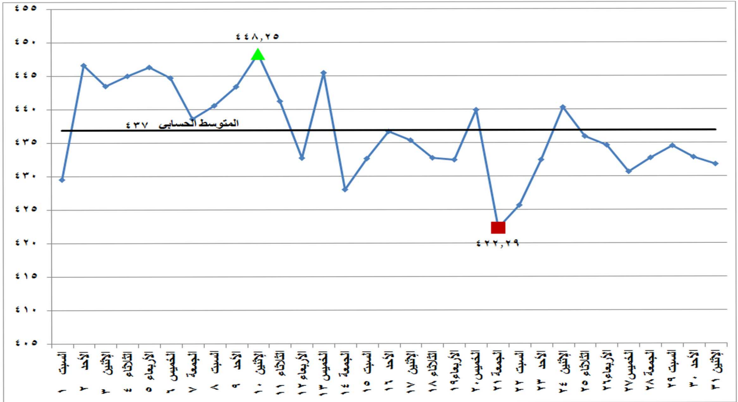
شكل (١٥) إجمالي الطاقة الكهربائية المنتجة من كل المصادر الأولية خلال شهر أغسطس ٢٠٢٠
