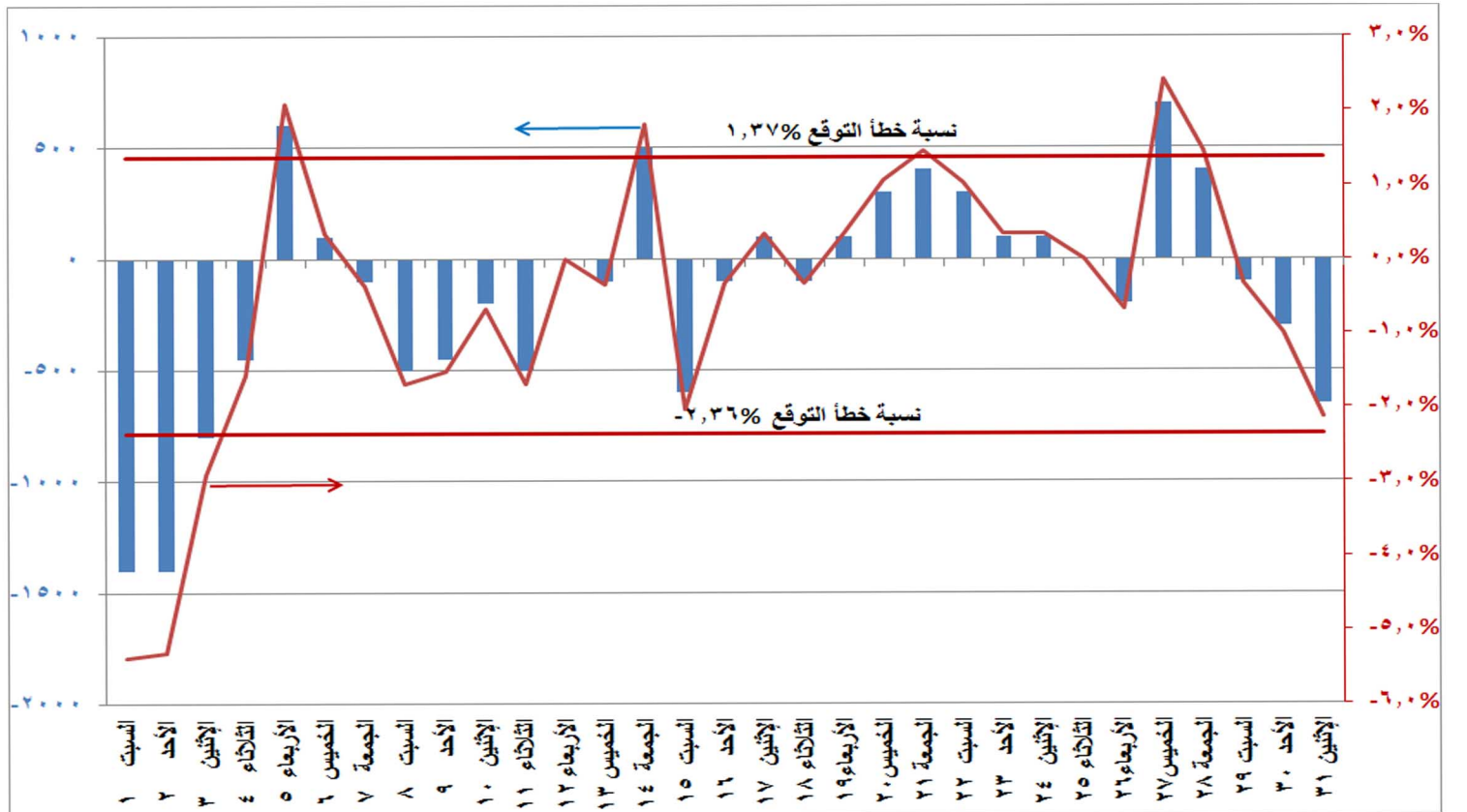
شكل (١٠) الفرق بين الحمل الأقصى المتوقع والمسجل فعليا ونسبة الفرق إلى الحمل المسجل فعليا خلال شهر أغسطس ٢٠٢٠
