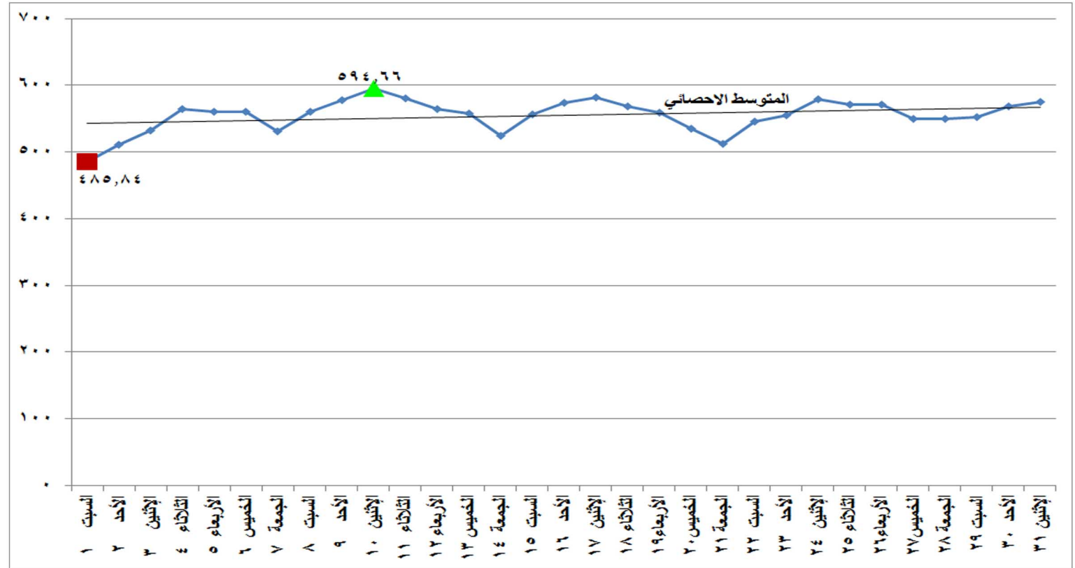
شكل (١٧) الطاقة الكهربائية المنتجة من الغاز الطبيعي خلال شهر أغسطس ٢٠٢٠
