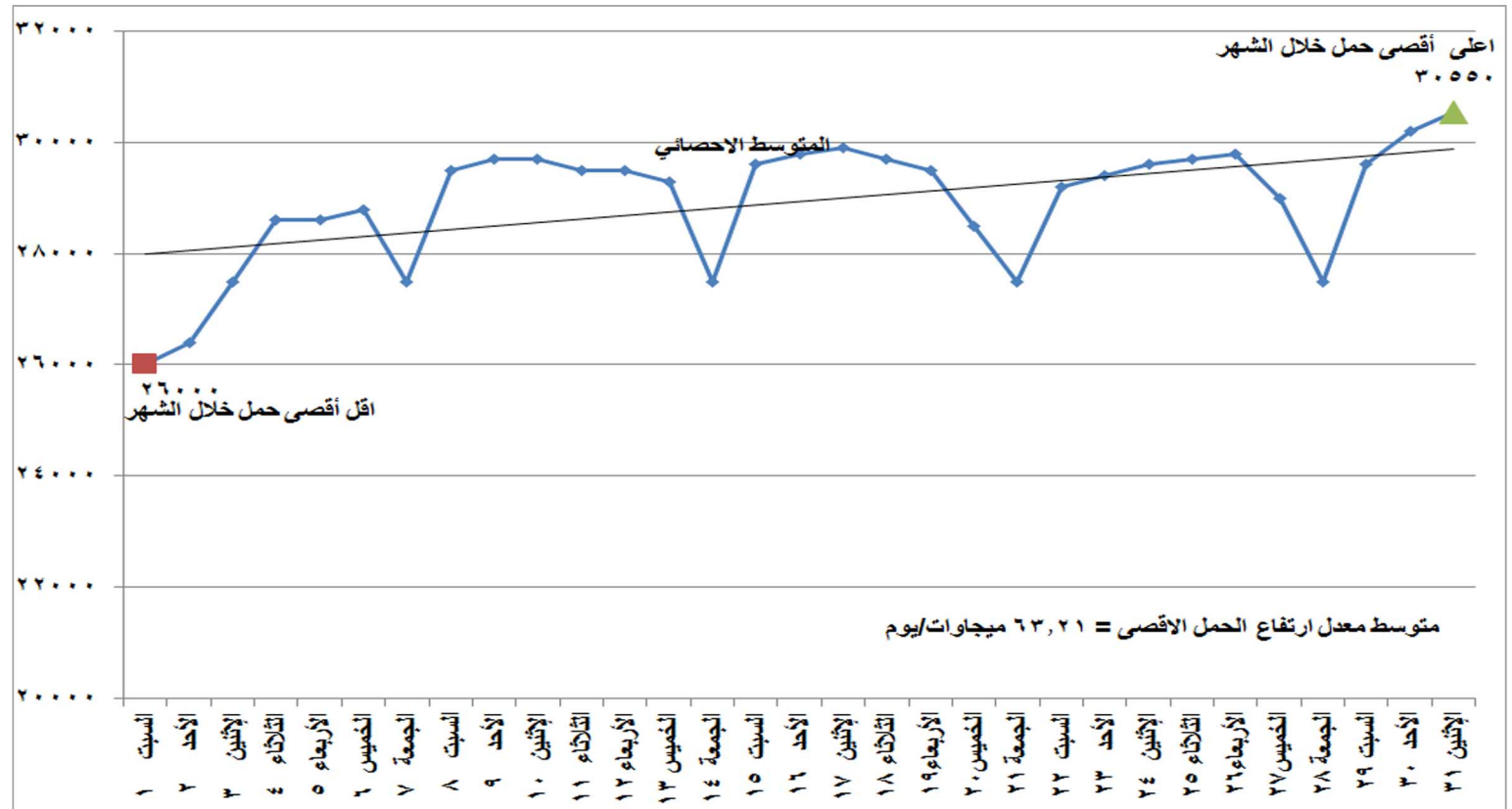
شكل (١) تطور الحمل الاقصى اليومي خلال شهر أغسطس ٢٠٢٠
