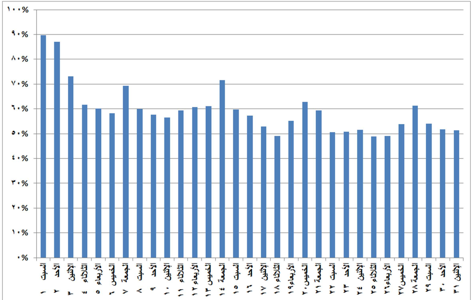
شكل (٢٨) نسب الفائض للحمل الاقصى المسجل يوميا خلال شهر أغسطس ٢٠٢٠
