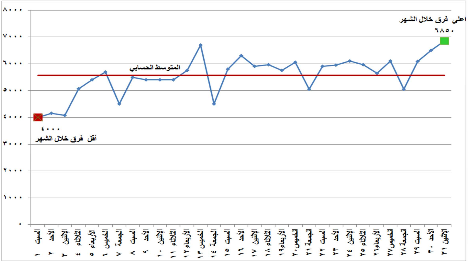
شكل (٣) الفرق بين أقصى وأدنى حمل خلال شهر أغسطس ٢٠٢٠
