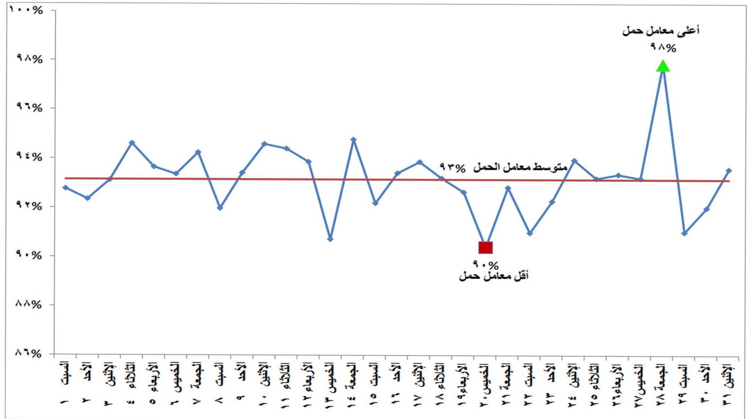
شكل (١٢) إجمالي معامل الحمل لوحدات الانتاج خلال شهر أغسطس ٢٠٢٠
