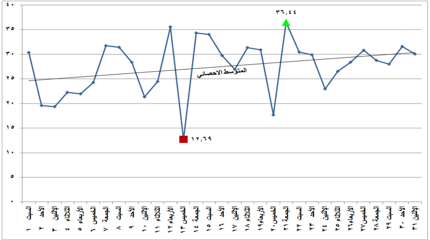
شكل (٢٥) الطاقة الكهربائية المنتجة من الرياح والشمس خلال شهر أغسطس ٢٠٢٠
