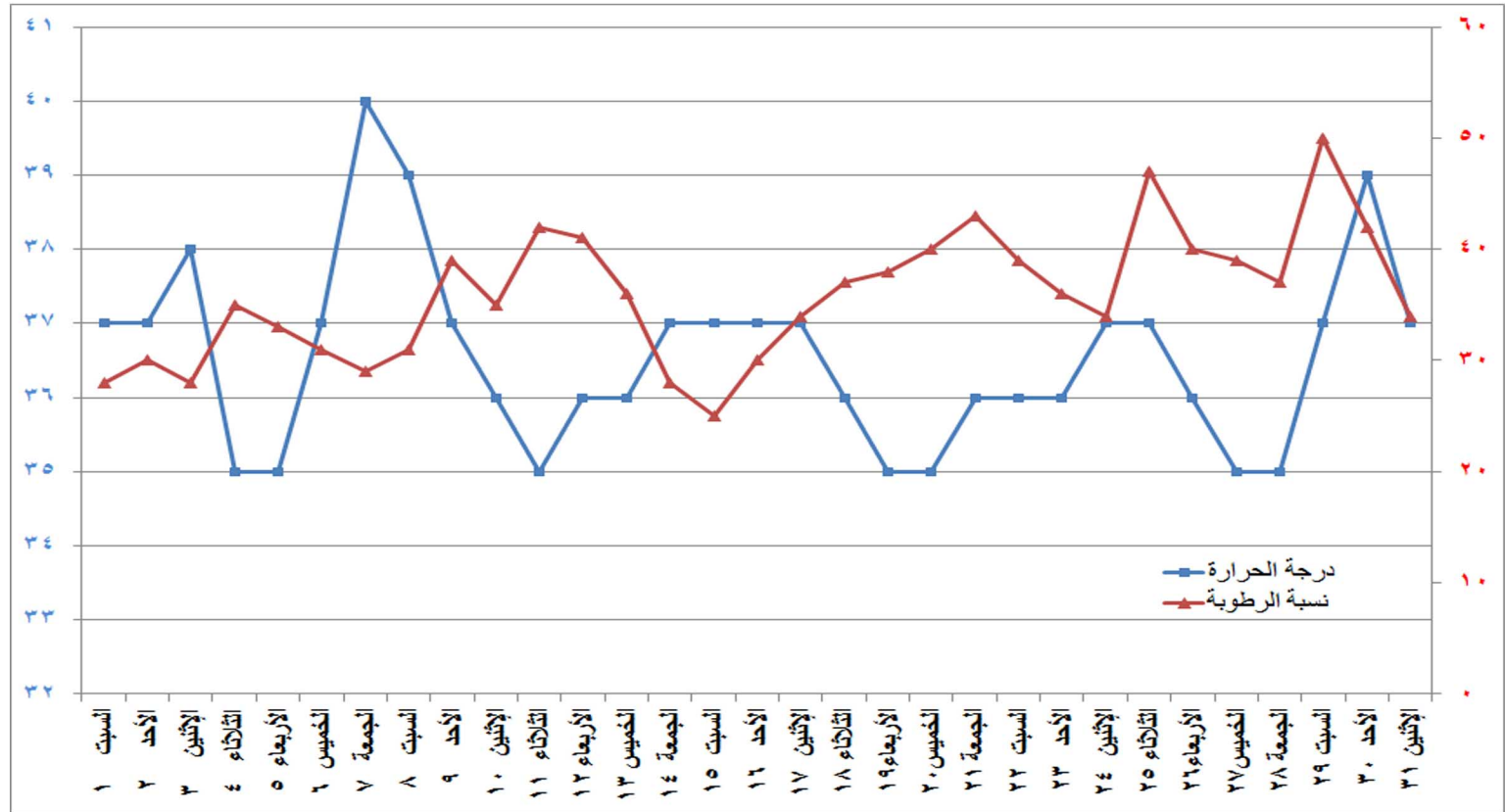
شكل (١١) التغيير في درجة الحرارة والرطوبة النسبية خلال شهر أغسطس ٢٠٢٠
