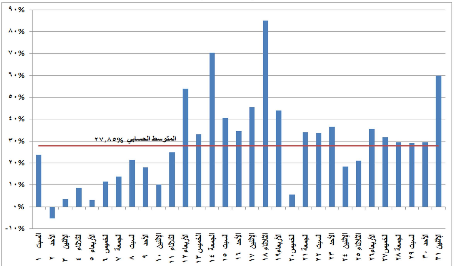
شكل (٢١) الطاقة الكهربائية المنتجة من المصادر غير الحرارية خلال شهر اغسطس ٢٠٢٠
